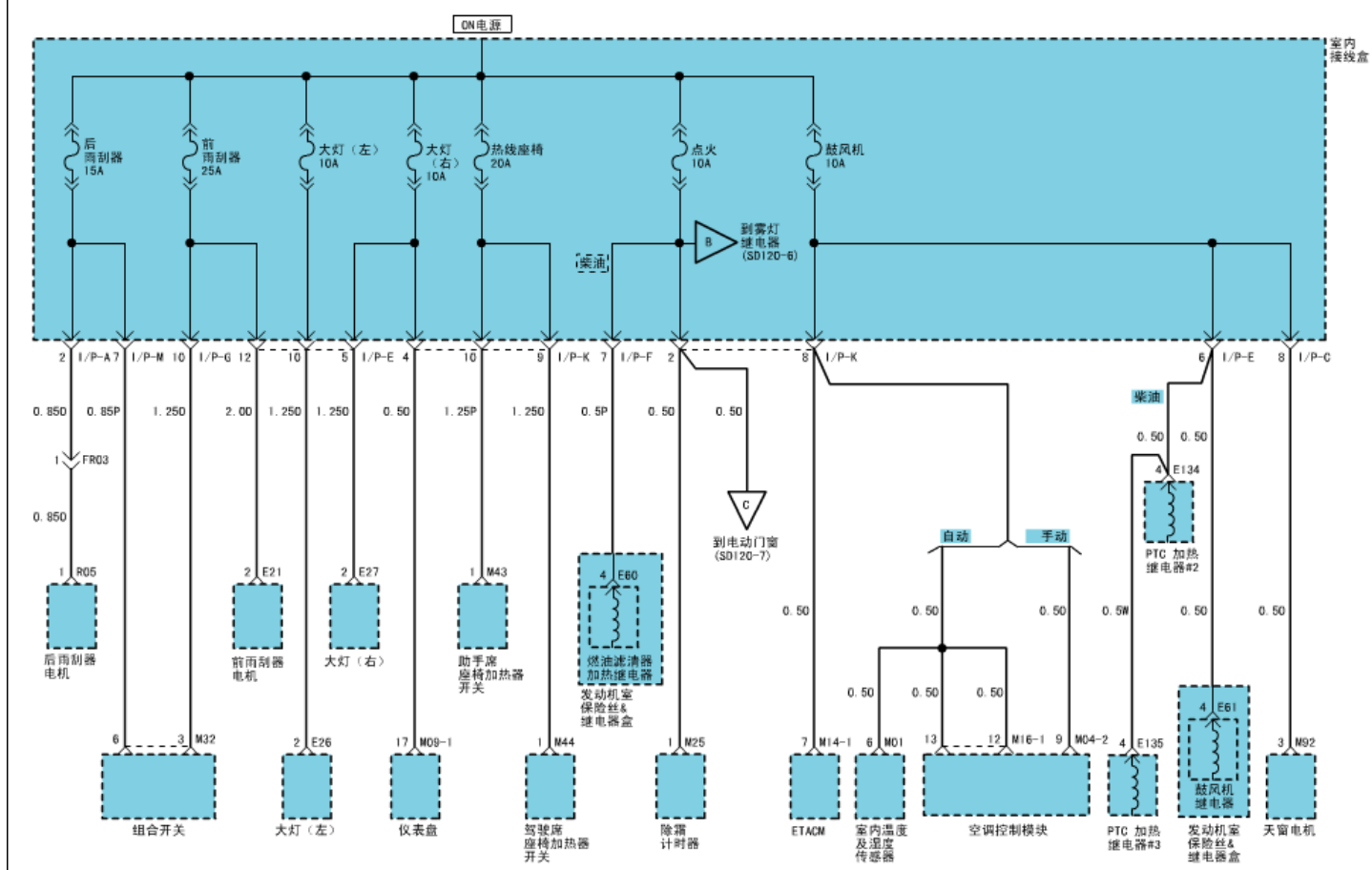
保險絲分布 (3)
